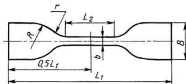
Рисунок 2 - Образец-лопатка типа 2
