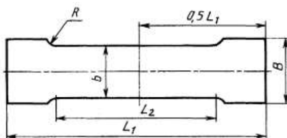
Рисунок 1 - Образец-лопатка типа 1
