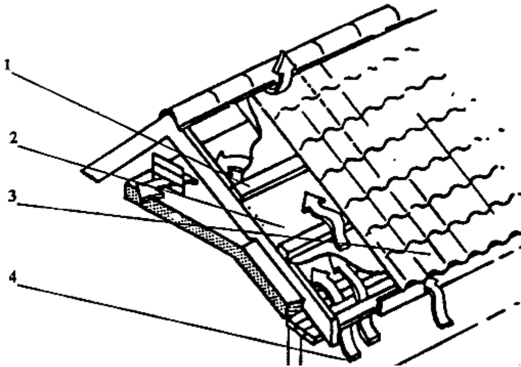
Рис.7. Движение воздуха от карниза к коньку 1- обрешетка; 2- гидроизоляционный рулонный материал; 3- металлочерепица; 4- направление движения воздуха
