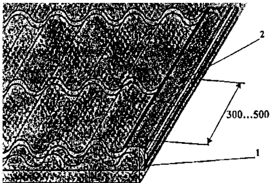
Рис.15. Крепление торцевой планки к деревянному основанию 1- торцевая планка; 2- винт самонарезающей
