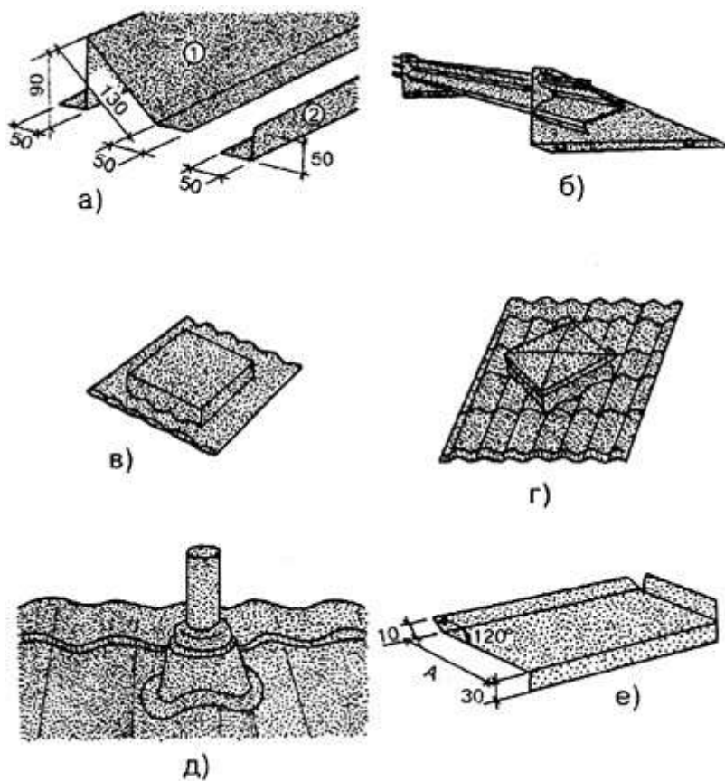
Рис.2 г. Комплектующие материалы для кровель из металлочерепицы и профнастила a - снегозадержатель, длина 2000 мм, на все типы профиля; б - снегозадержатель, длина 300 мм, на все типы профиля; в - панель для сквозного выхода 400x400; г - пожарный люк; д - панель с выходным отверстием, тип Б; е -лист для покрытия наружных углублений, длина 2000 мм, на все типы профиля
