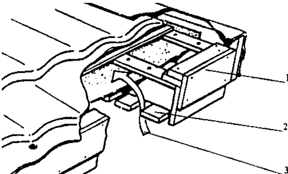
Рис.8. Карнизный участок крыши 1- защитная доска; 2- зашивка карниза; 3- направление движения воздуха
