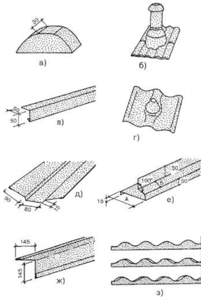
Рис.2 б. Комплектующие материалы для кровель из металлочерепицы и профнастила a - конец на коньковую планку; б - выходная труба; в -торцевая планка 50x50, длина 2000 мм, на все типы профиля; г - панель с выходным отверстием; д - планка для внутренних швов и стыков, на все типы профиля; е - верхняя планка, длина 2000 мм, на все типы профиля; ж - планка для внутренних углов, длина 2000 мм, на все типы профиля; з - уплотнения, особые для каждого профиля
