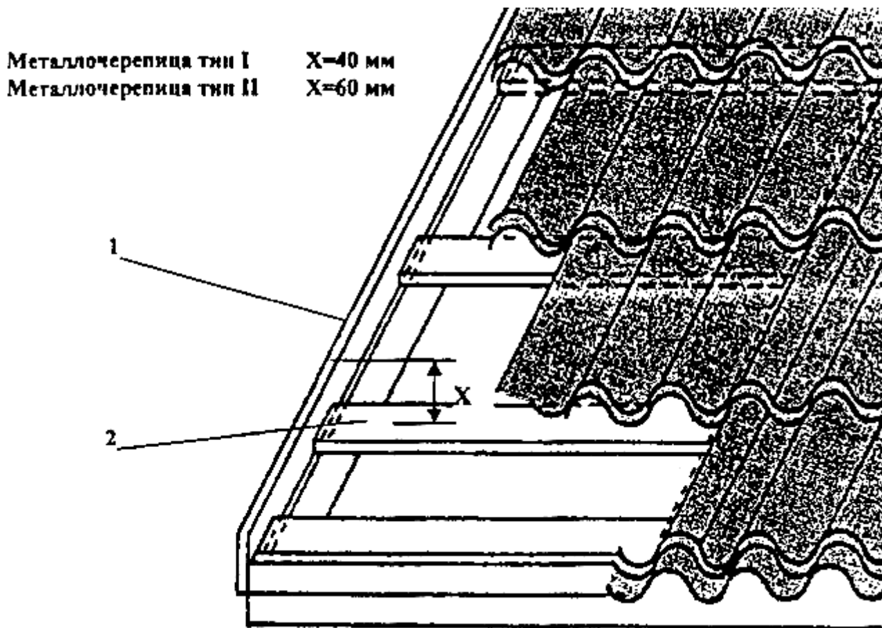
Рис.9. Размещение торцевой планки 1- торцевая планка; 2- обрешетка
